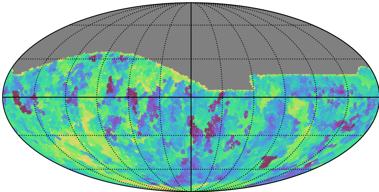
all_long_v3.4_10yrs All sky i band: Min saturation_mag
