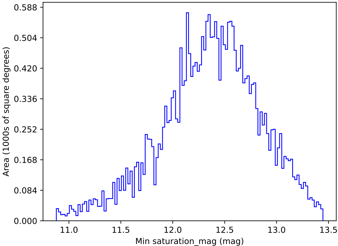
all_long_v3.4_10yrs All sky i band: Min saturation_mag
