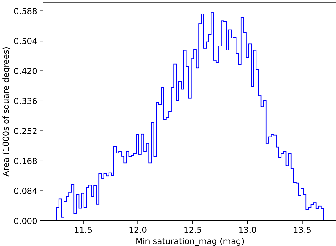
all_long_v3.4_10yrs All sky g band: Min saturation_mag
