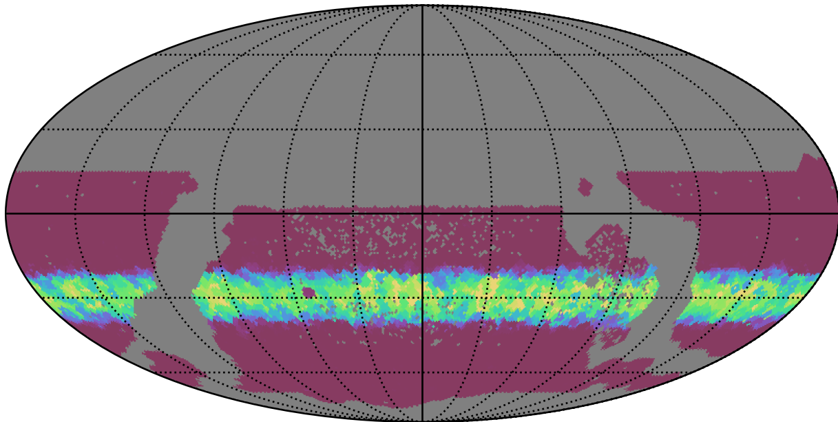
all_long_v3.4_10yrs WFD z band: Min normairmass
