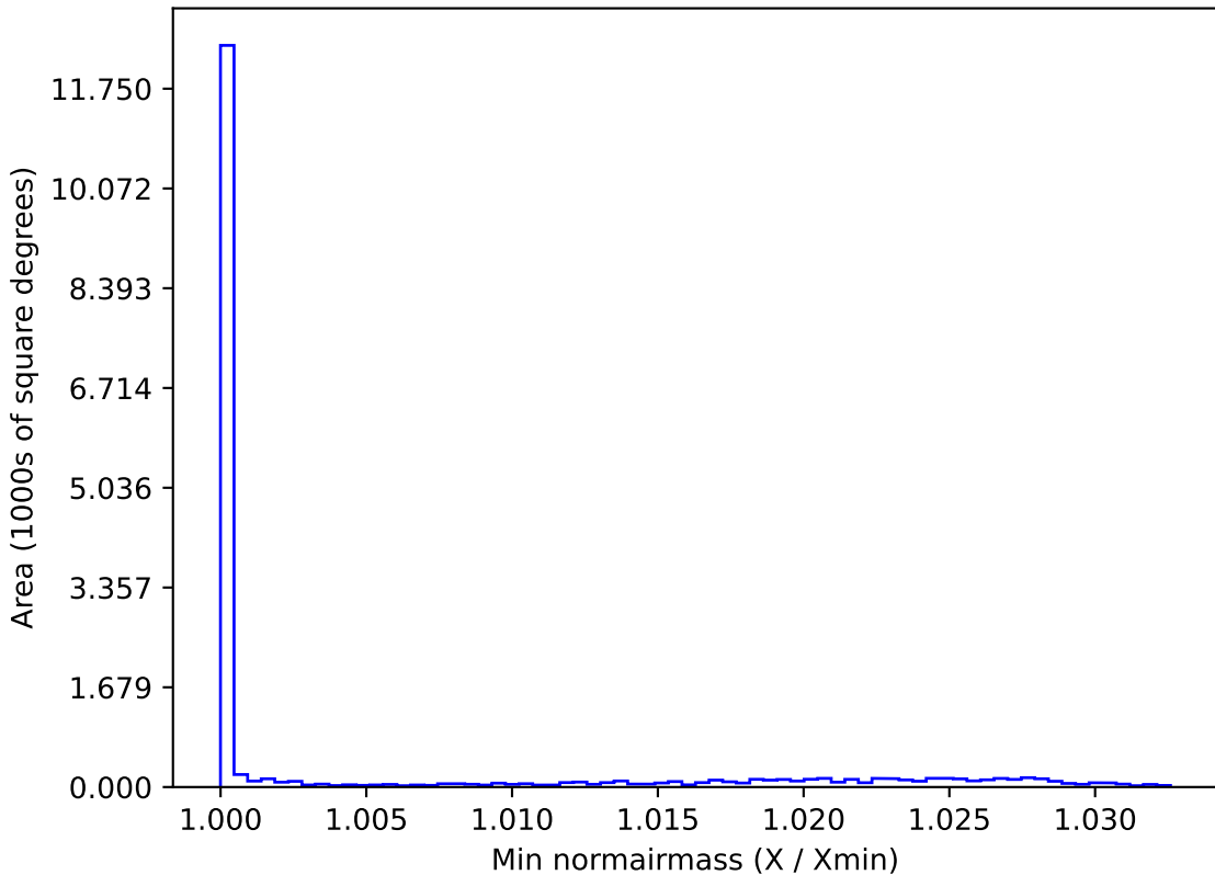
all_long_v3.4_10yrs WFD z band: Min normairmass
