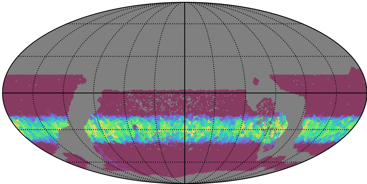
all_long_v3.4_10yrs WFD u band: Min normairmass
