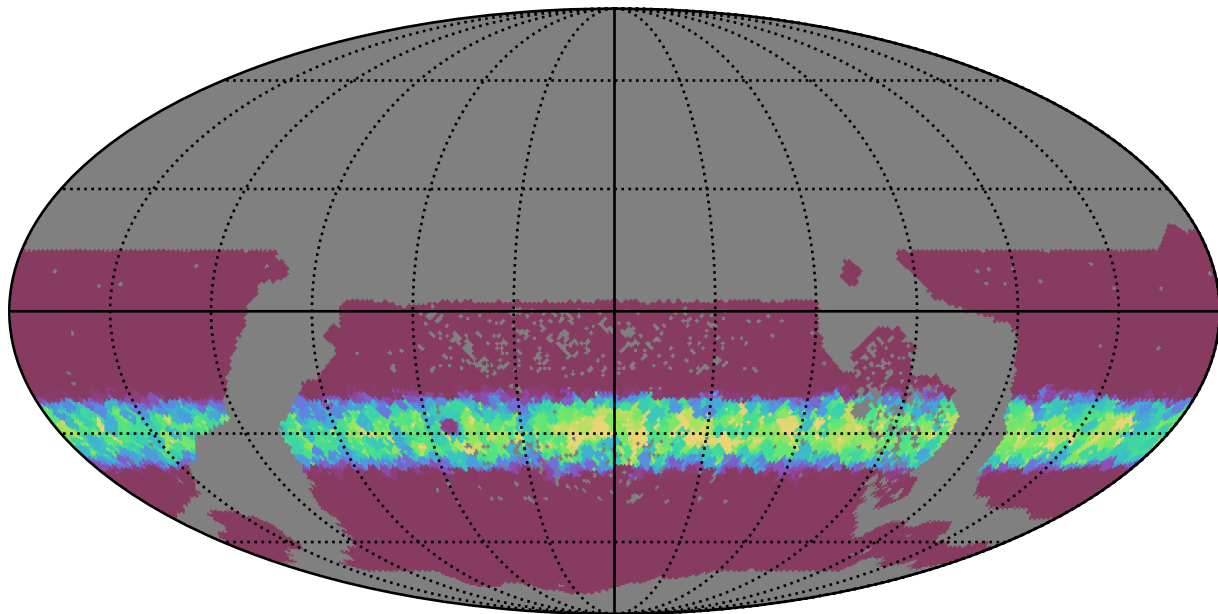
all_long_v3.4_10yrs WFD r band: Min normairmass
