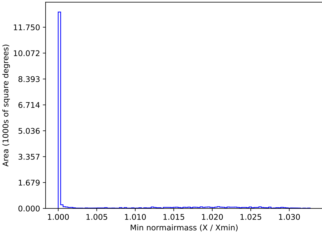
all_long_v3.4_10yrs WFD r band: Min normairmass
