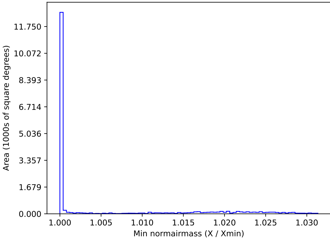
all_long_v3.4_10yrs WFD i band: Min normairmass
