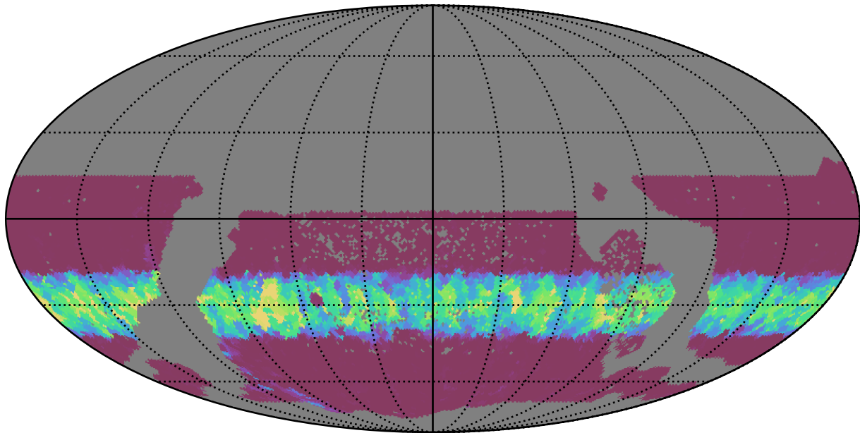
all_long_v3.4_10yrs WFD g band: Min normairmass
