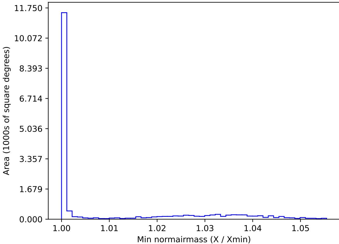
all_long_v3.4_10yrs WFD g band: Min normairmass
