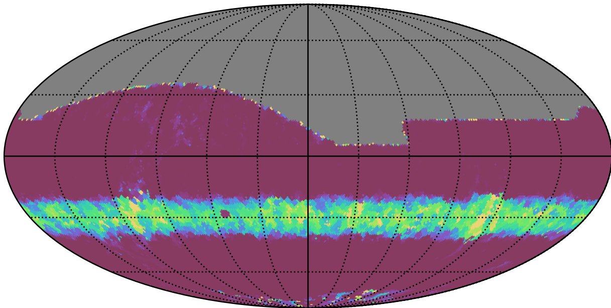
all_long_v3.4_10yrs All sky z band: Min normairmass
