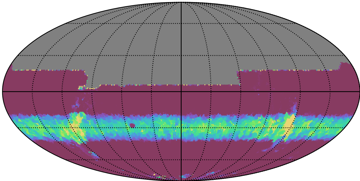
all_long_v3.4_10yrs All sky y band: Min normairmass
