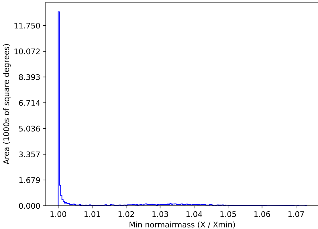
all_long_v3.4_10yrs All sky u band: Min normairmass
