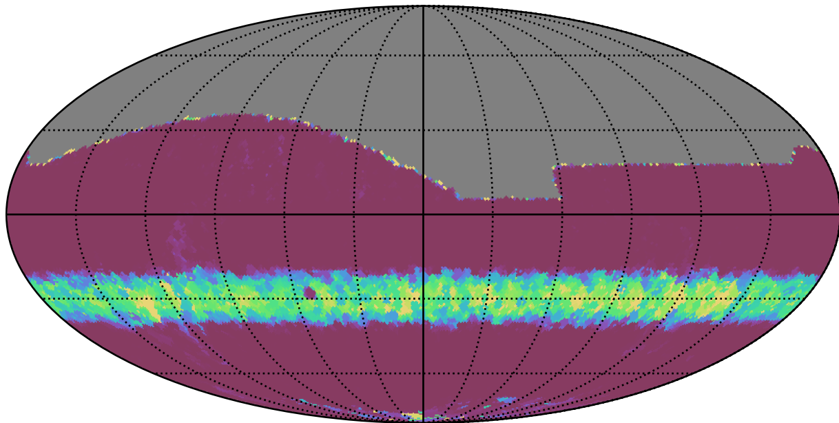
all_long_v3.4_10yrs All sky i band: Min normairmass
