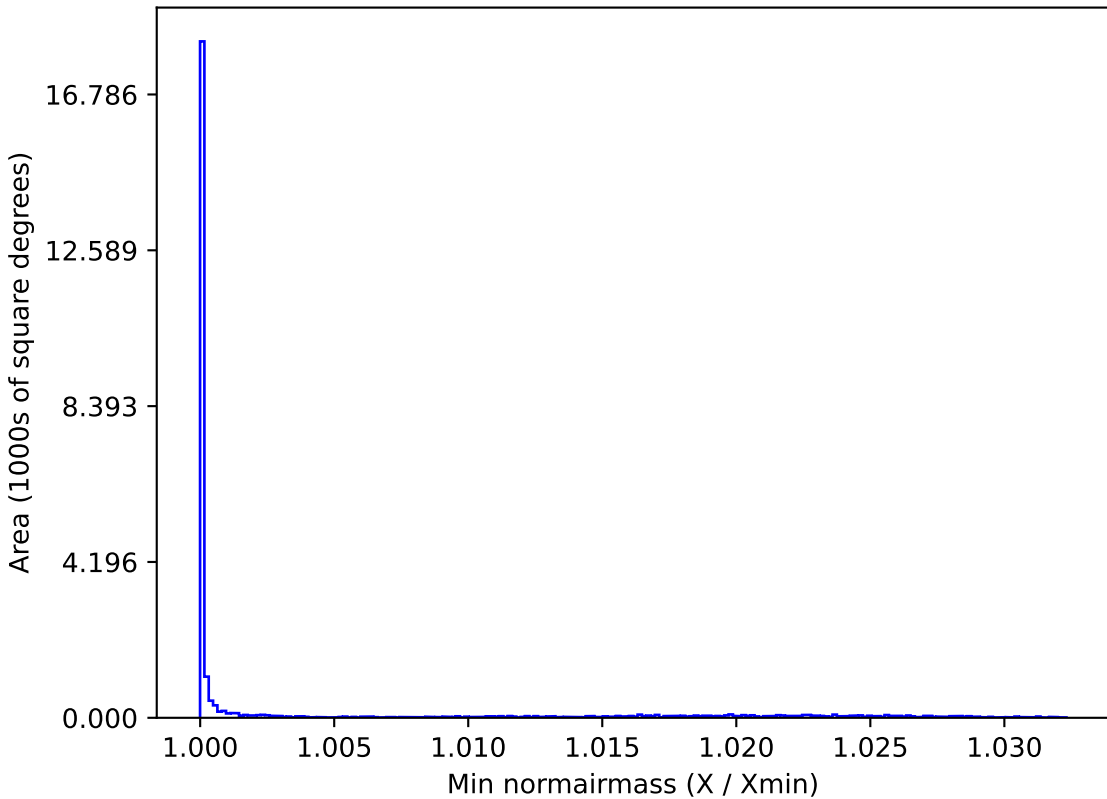
all_long_v3.4_10yrs All sky i band: Min normairmass
