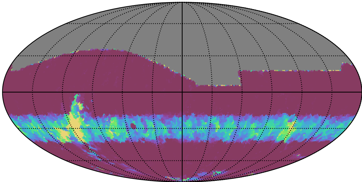
all_long_v3.4_10yrs All sky g band: Min normairmass
