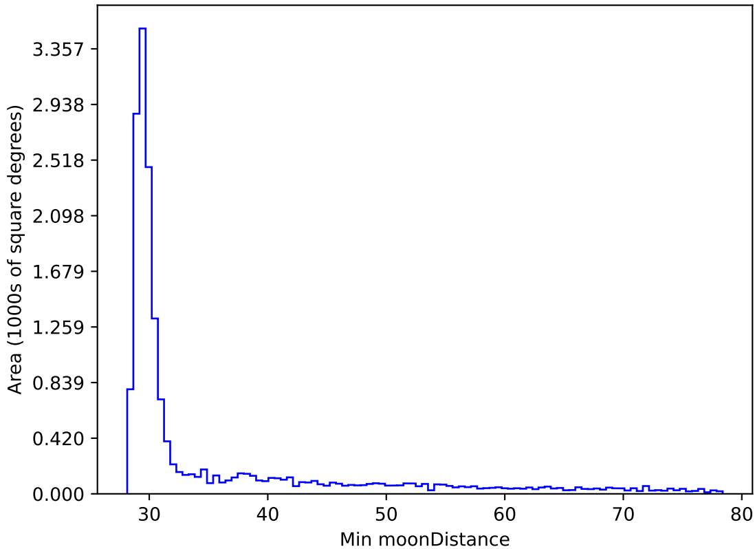
all_long_v3.4_10yrs WFD y band: Min moonDistance
