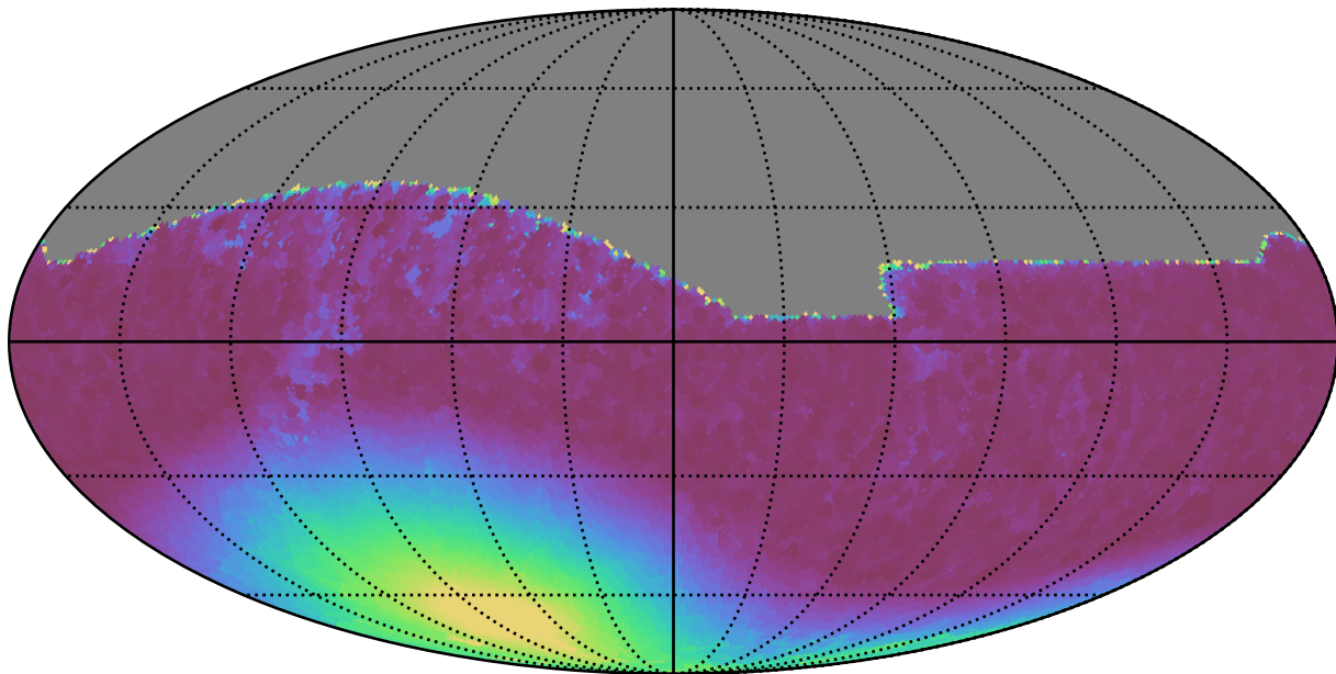
all_long_v3.4_10yrs All sky i band: Min moonDistance
