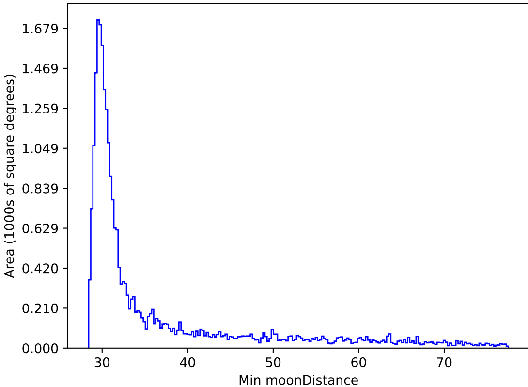
all_long_v3.4_10yrs All sky i band: Min moonDistance
