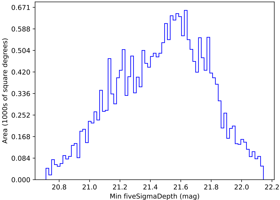
all_long_v3.4_10yrs Yr 1 y band: Min fiveSigmaDepth
