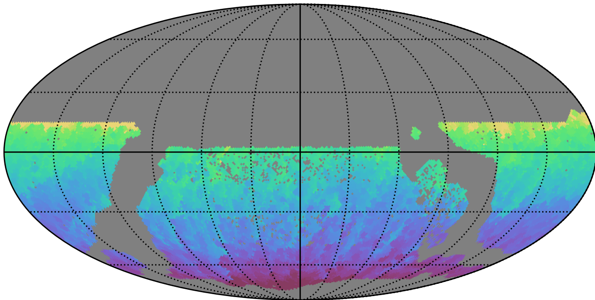
all_long_v3.4_10yrs WFD z band: Min HA
