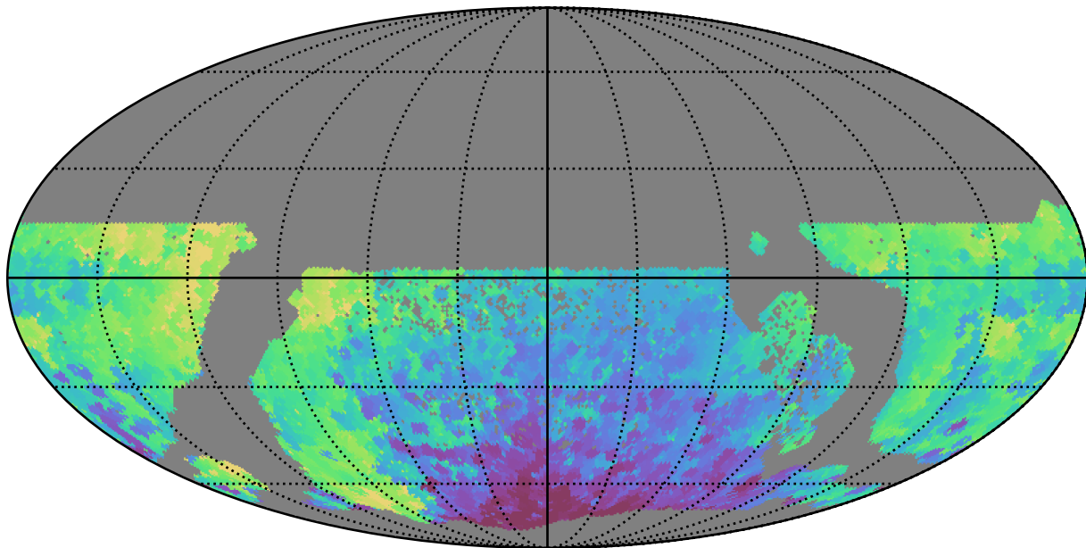
all_long_v3.4_10yrs WFD y band: Min HA
