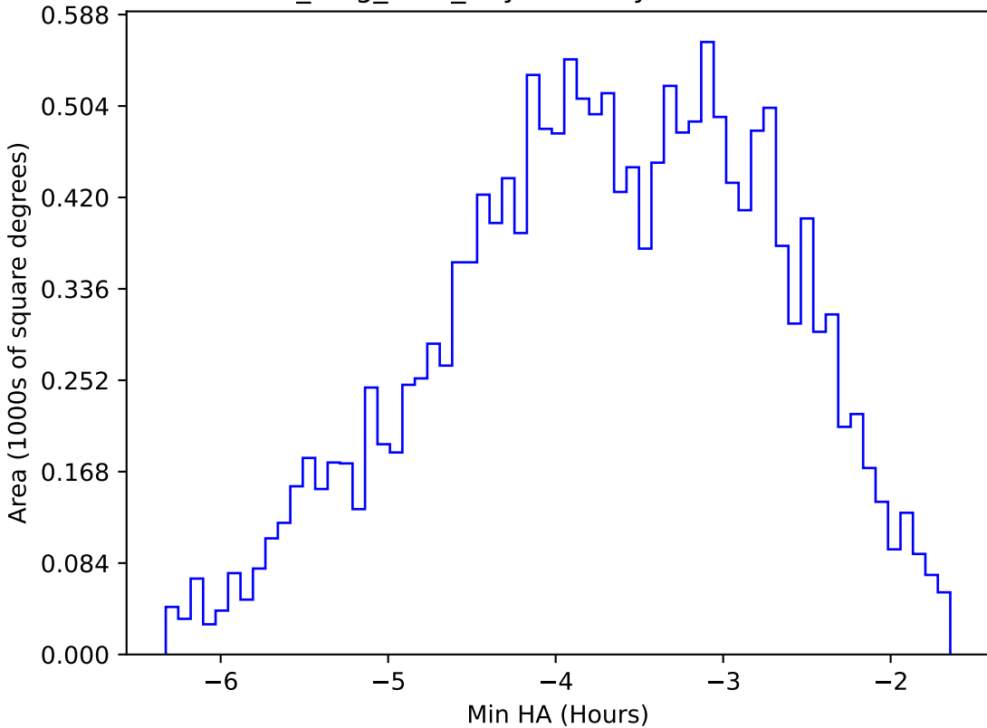
all_long_v3.4_10yrs WFD y band: Min HA
