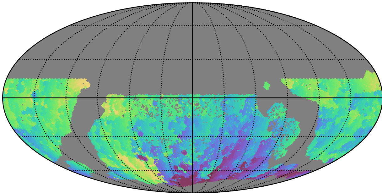
all_long_v3.4_10yrs WFD u band: Min HA
