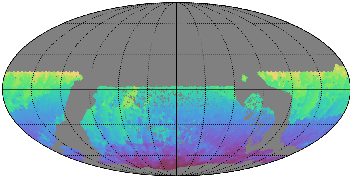
all_long_v3.4_10yrs WFD r band: Min HA
