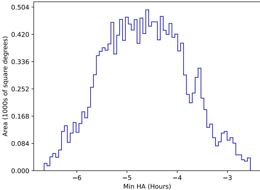
all_long_v3.4_10yrs WFD r band: Min HA
