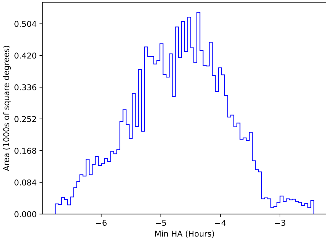
all_long_v3.4_10yrs WFD i band: Min HA
