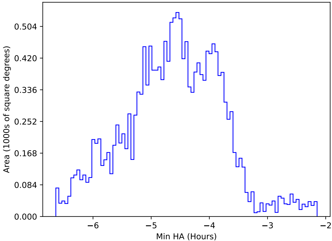
all_long_v3.4_10yrs WFD g band: Min HA
