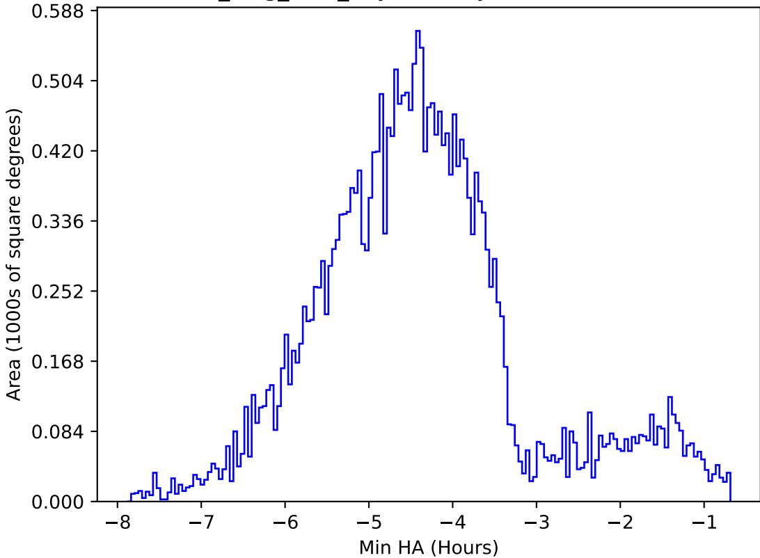
all_long_v3.4_10yrs All sky z band: Min HA
