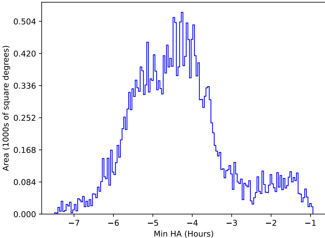
all_long_v3.4_10yrs All sky r band: Min HA
