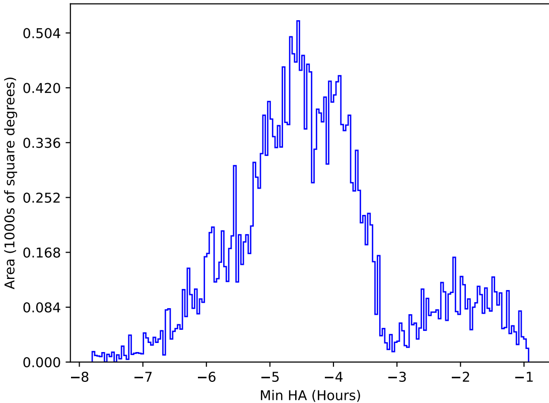
all_long_v3.4_10yrs All sky g band: Min HA
