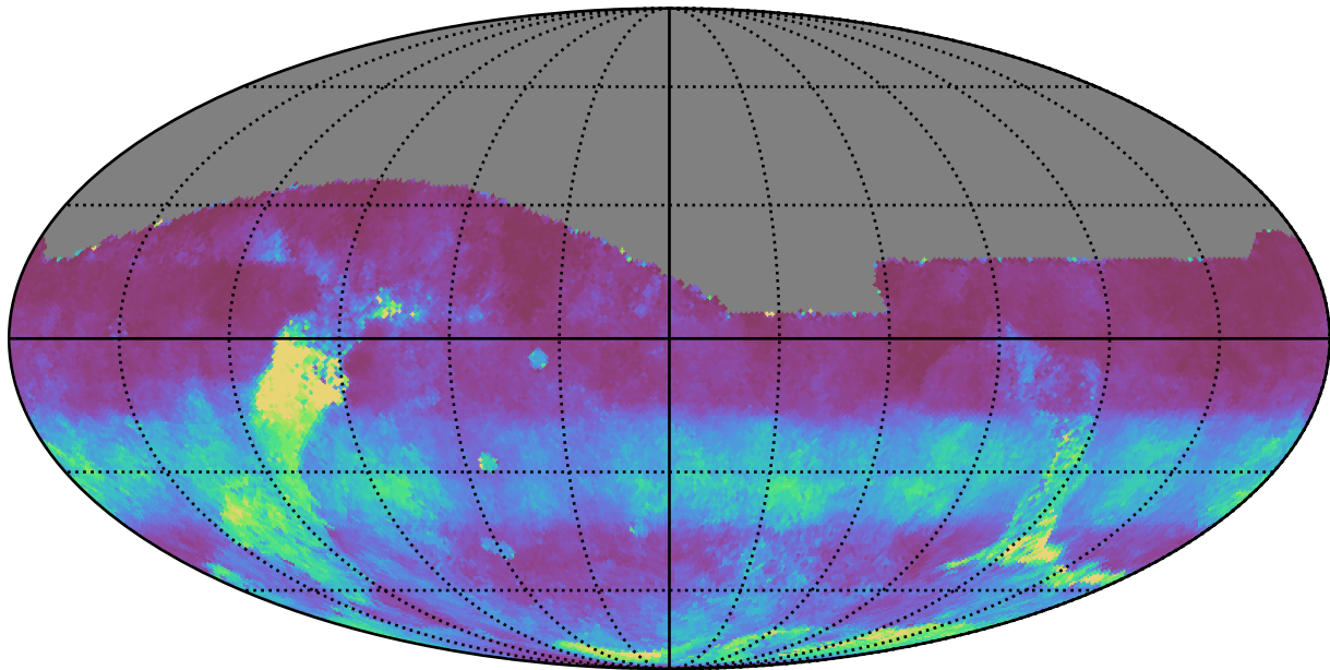
all_long_v3.4_10yrs All sky i band: Median normairmass
