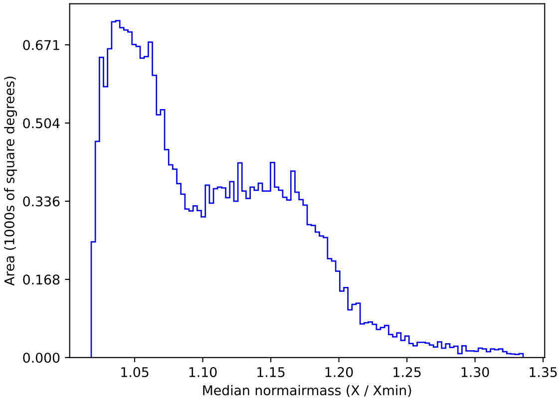
all_long_v3.4_10yrs All sky i band: Median normairmass
