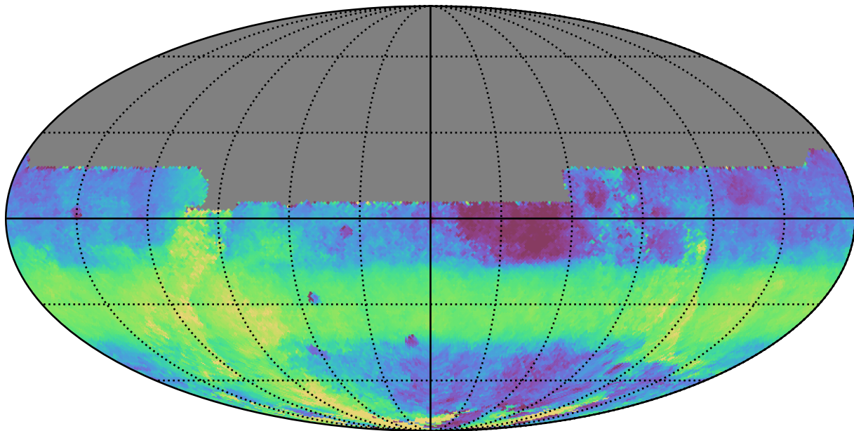
all_long_v3.4_10yrs All sky y band: Median HA
