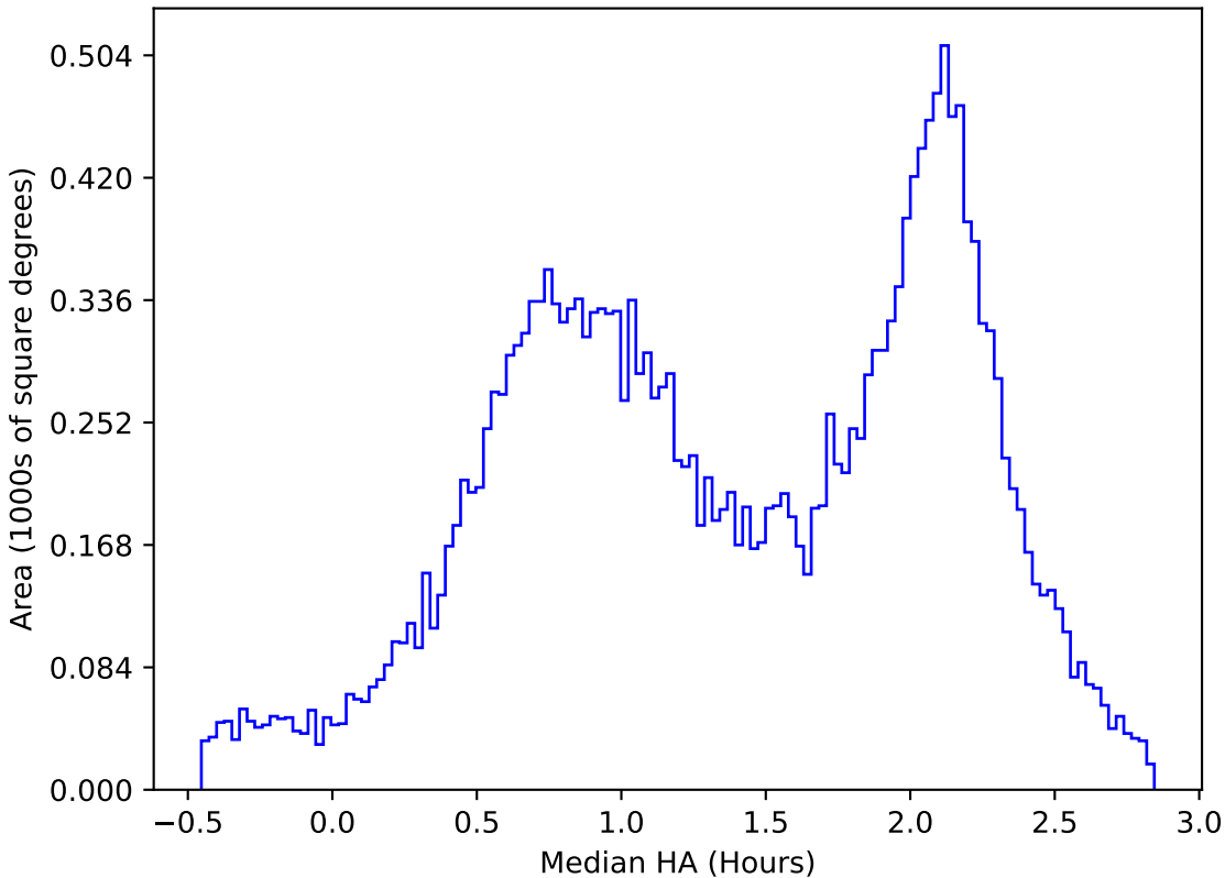
all_long_v3.4_10yrs All sky y band: Median HA
