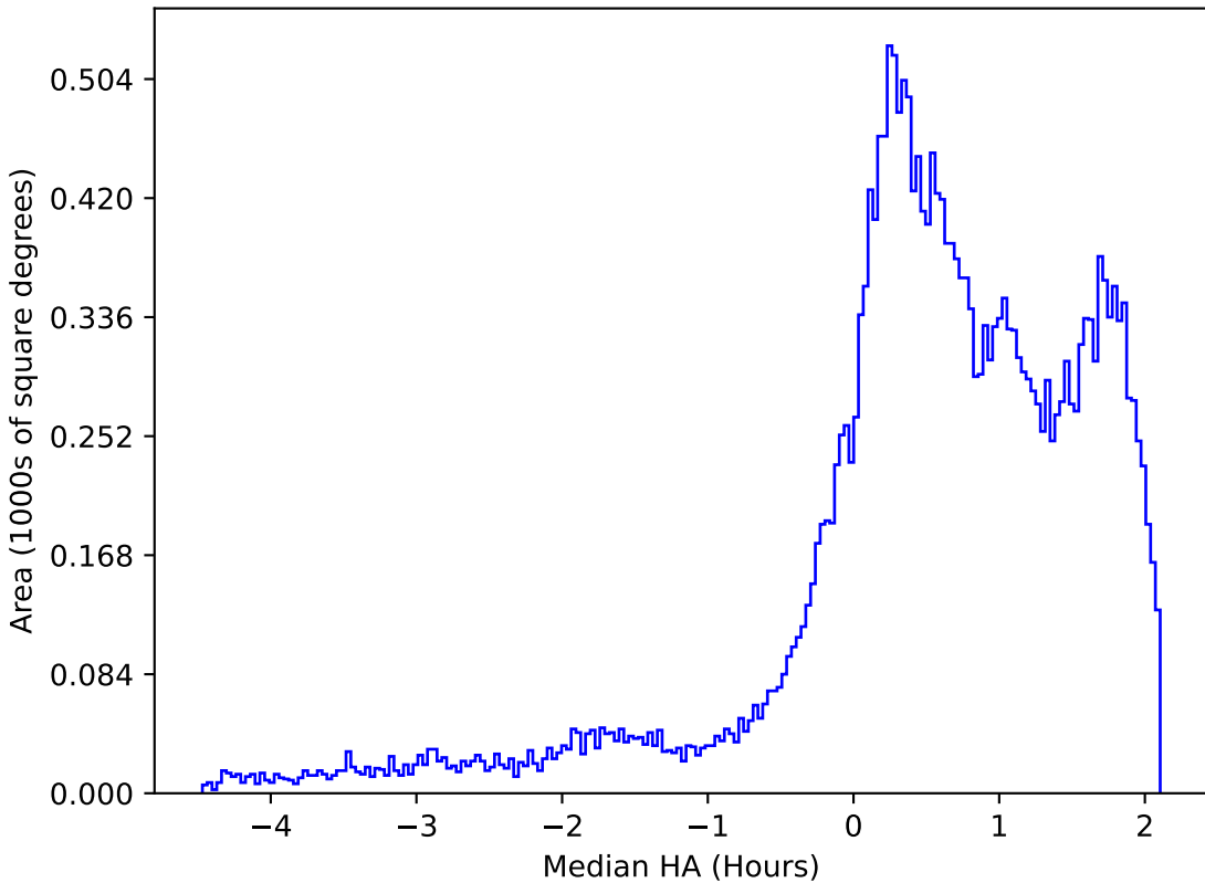
all_long_v3.4_10yrs All sky i band: Median HA
