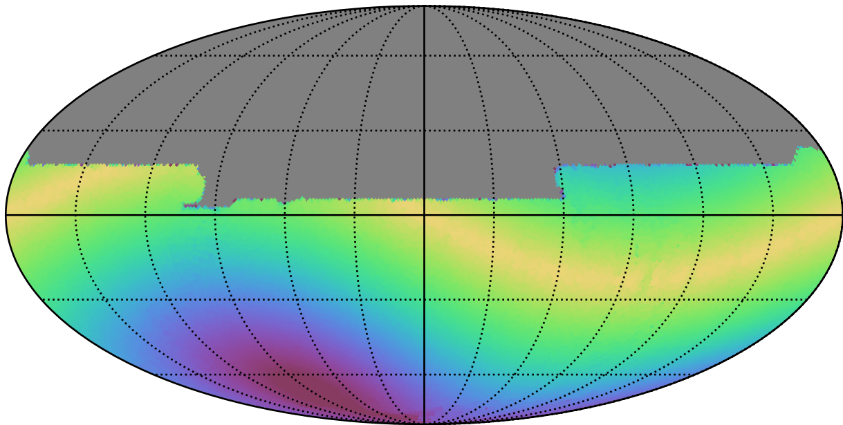
all_long_v3.4_10yrs All sky y band: Max solarElong
