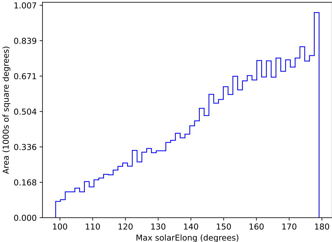
all_long_v3.4_10yrs All sky y band: Max solarElong
