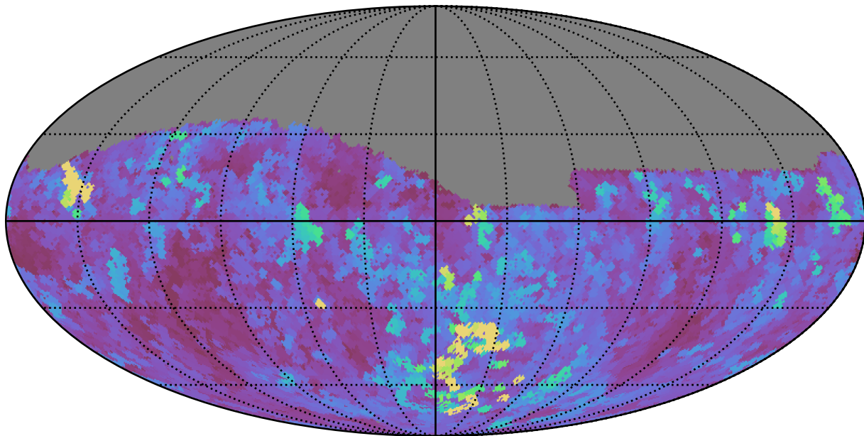
all_long_v3.4_10yrs Yr 1 z band: Max seeingGeom
