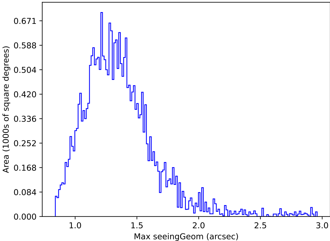
all_long_v3.4_10yrs Yr 1 z band: Max seeingGeom
