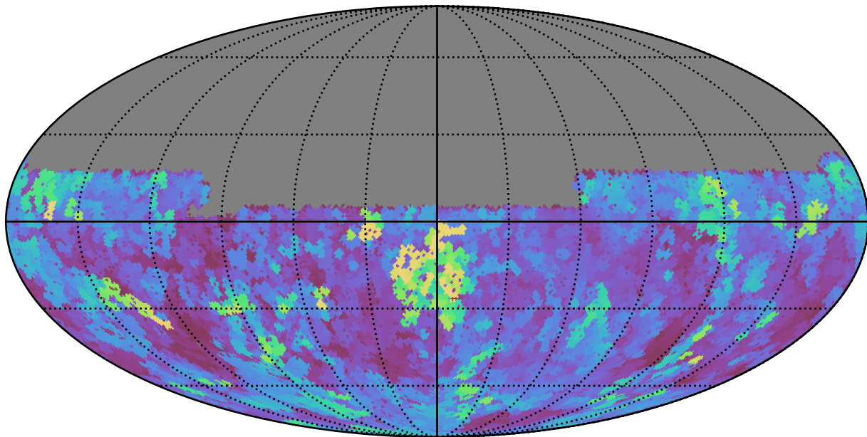
all_long_v3.4_10yrs Yr 1 y band: Max seeingGeom
