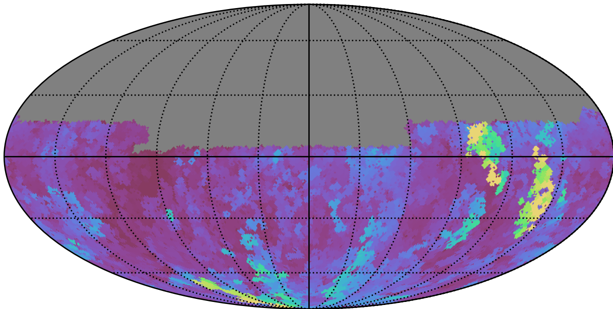
all_long_v3.4_10yrs Yr 1 u band: Max seeingGeom
