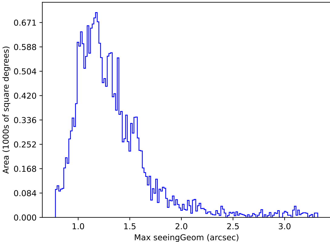
all_long_v3.4_10yrs Yr 1 u band: Max seeingGeom
