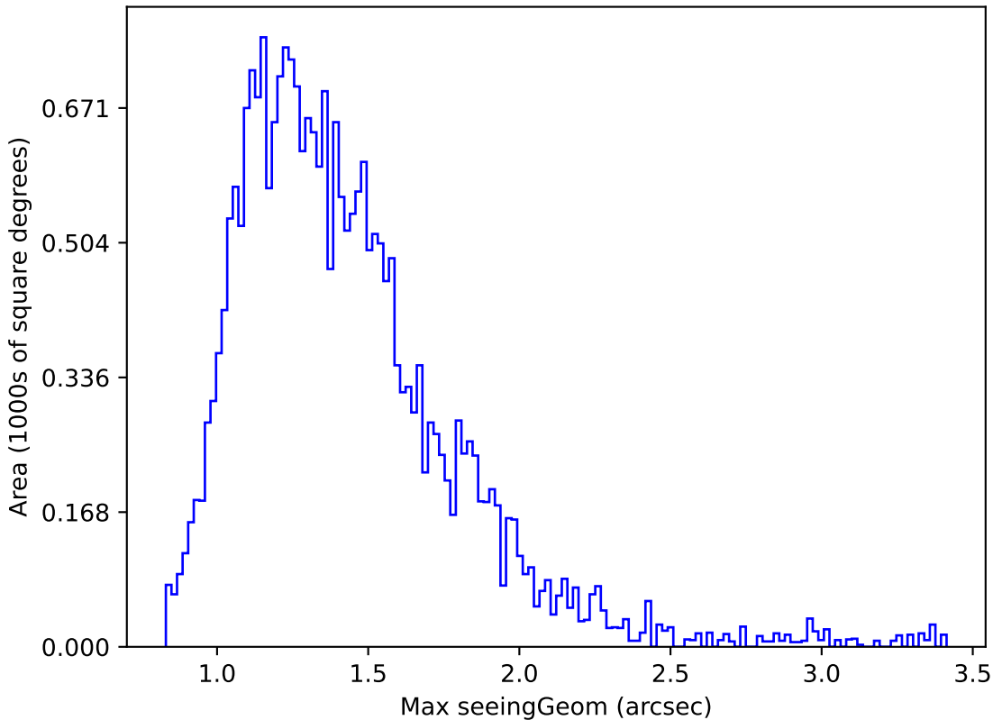
all_long_v3.4_10yrs Yr 1 g band: Max seeingGeom
