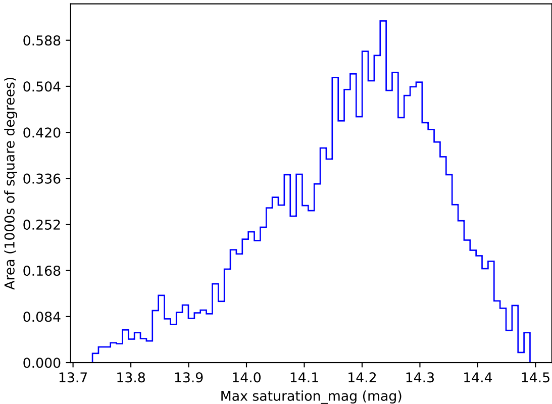
all_long_v3.4_10yrs WFD y band: Max saturation_mag
