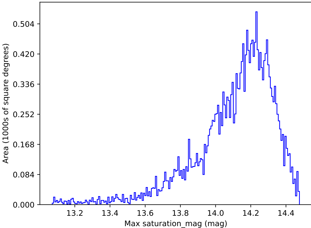
all_long_v3.4_10yrs All sky y band: Max saturation_mag
