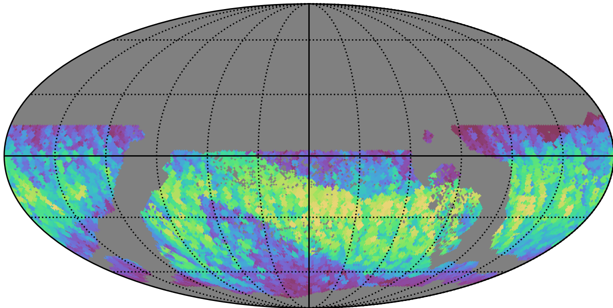
all_long_v3.4_10yrs WFD z band: Max normairmass
