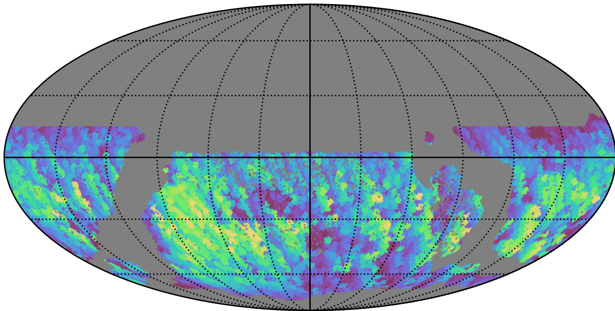
all_long_v3.4_10yrs WFD y band: Max normairmass
