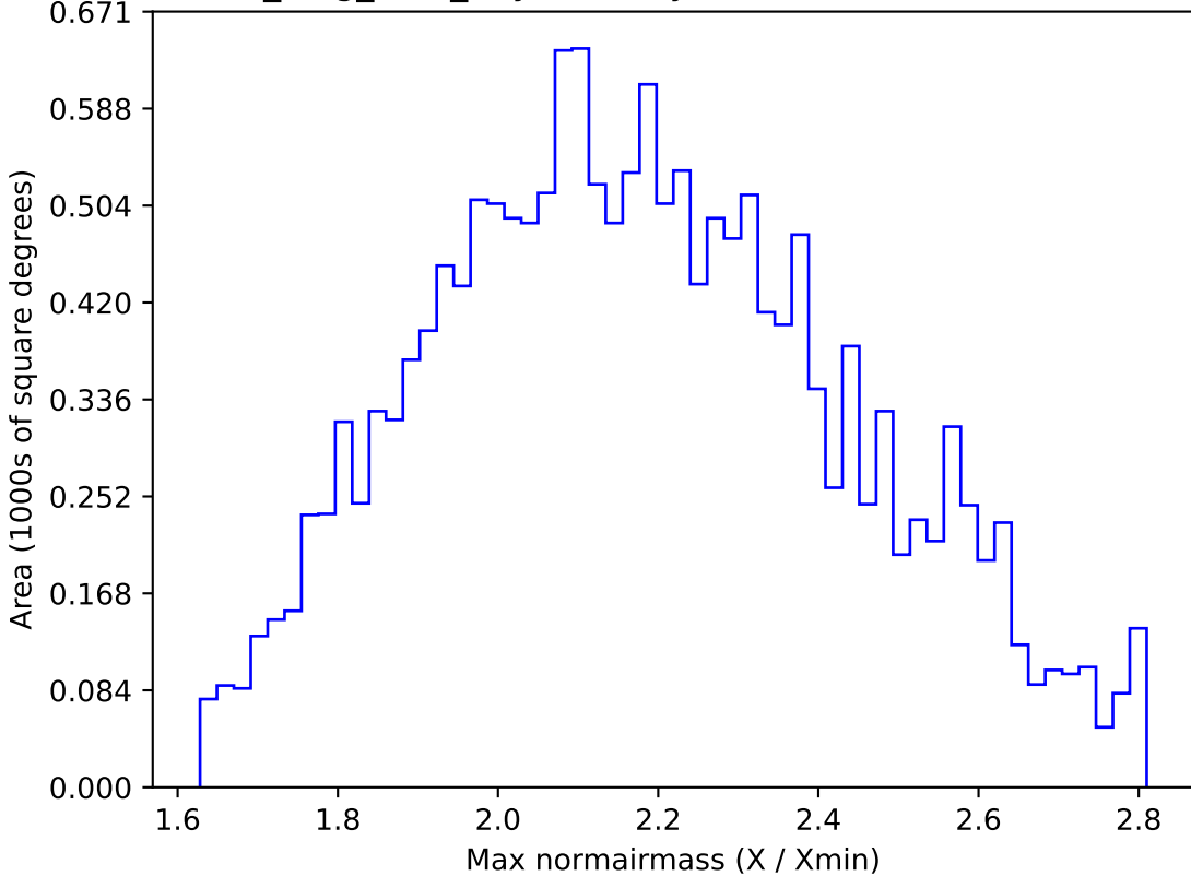
all_long_v3.4_10yrs WFD y band: Max normairmass
